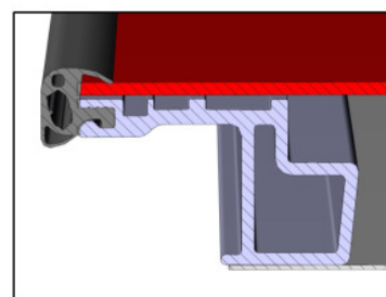
SEZIONE B-B SECTION B-B
