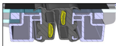
SEZIONE C-C SECTION C-C
