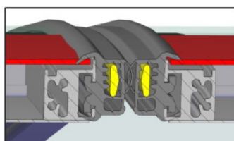
SEZIONE A-A SECTION A-A
