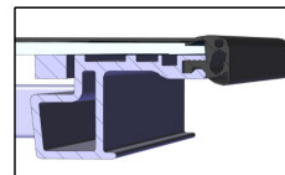
SEZIONE D-D SECTION D-D
