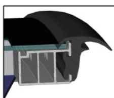
SEZIONE B-B SECTION B-B
