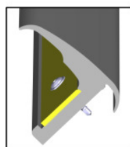
SEZIONE Z-Z SECTION Z-Z
