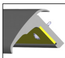
SEZIONE X-X SECTION X-X
