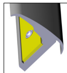
VISTA DA W VIEW W
