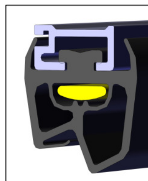
SEZIONE Y-Y SECTION Y-Y
