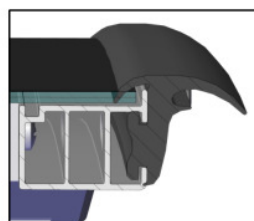
SEZIONE E-E SECTION E-E
